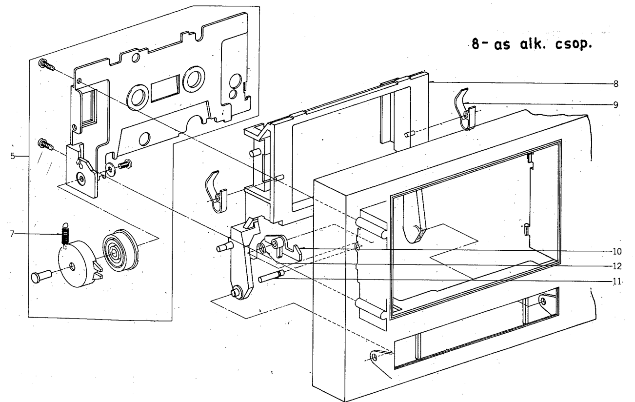
KAZETTA-AJTÓ MECHANIZMUSA
